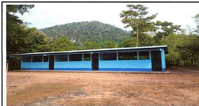
Foto 6: Instalacion de Canales con bajas de aguas pluvial.
